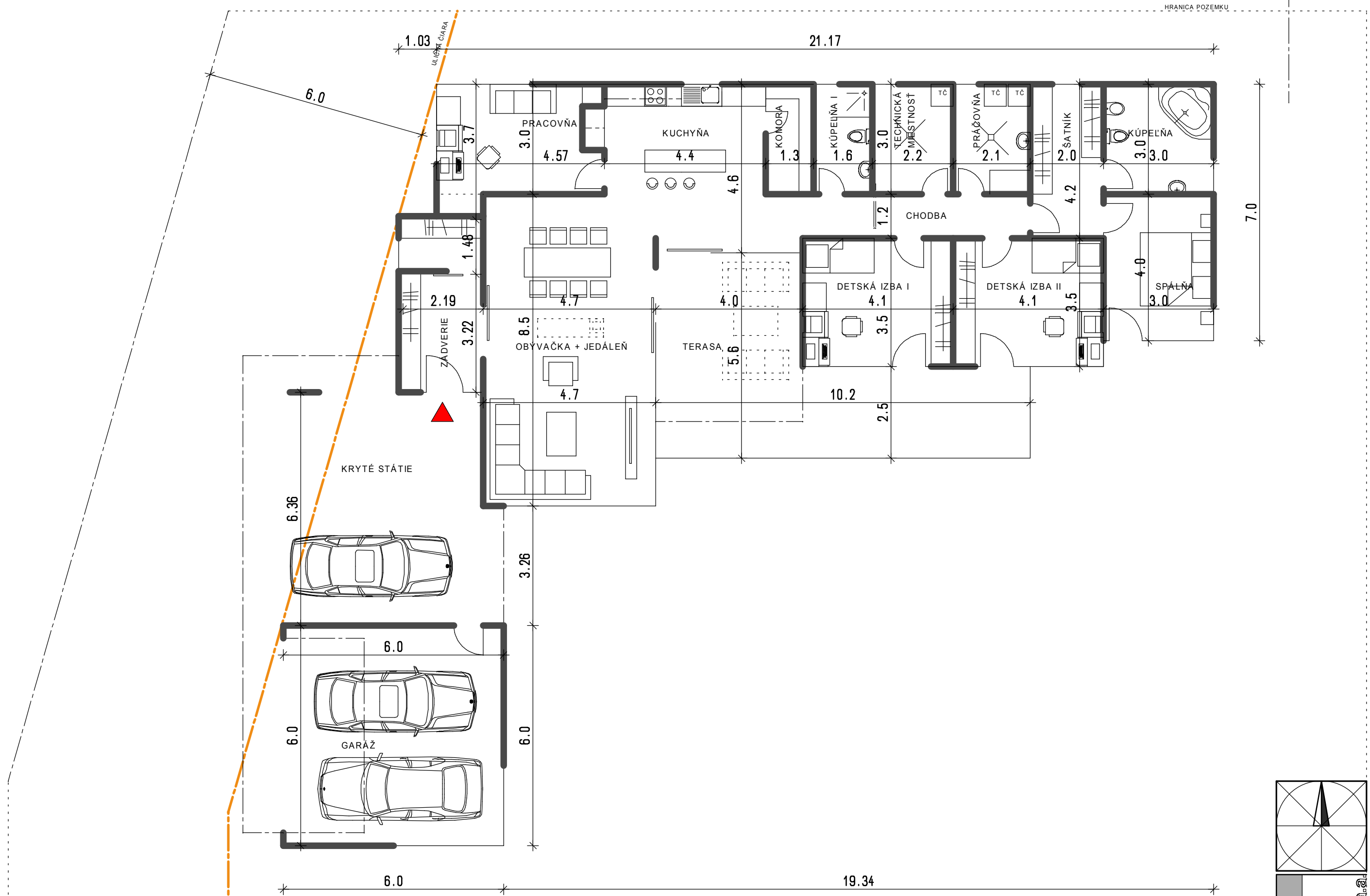
RD DANIŠ - HÔRKY M1:100 - PÔDORYS 1.NP - 170M2 + TERASA + GARÁŽ
